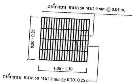
ฝาบ่อพักเหล็ก
